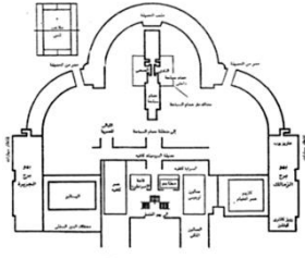
شكل (١٢/٢٢) مستطد أفقي الدور الأرضي - فندق ماريوت القاهرة - يظهر فيه أماكن الطاقم والخدمات وهو برج الريفليك ويندوز برج الجزيرة والأستاد الخلفي الدائري ومنطقة حمام السباحة والإضافات الملحقة للقصر (المصدر: فندق ماريوت)
